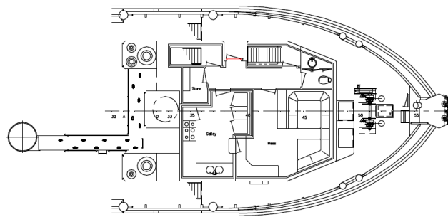
Maindeck
