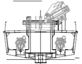
WEB FRAME 18
