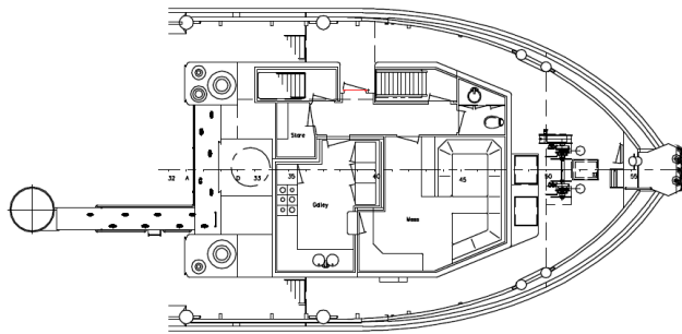
Maindeck
